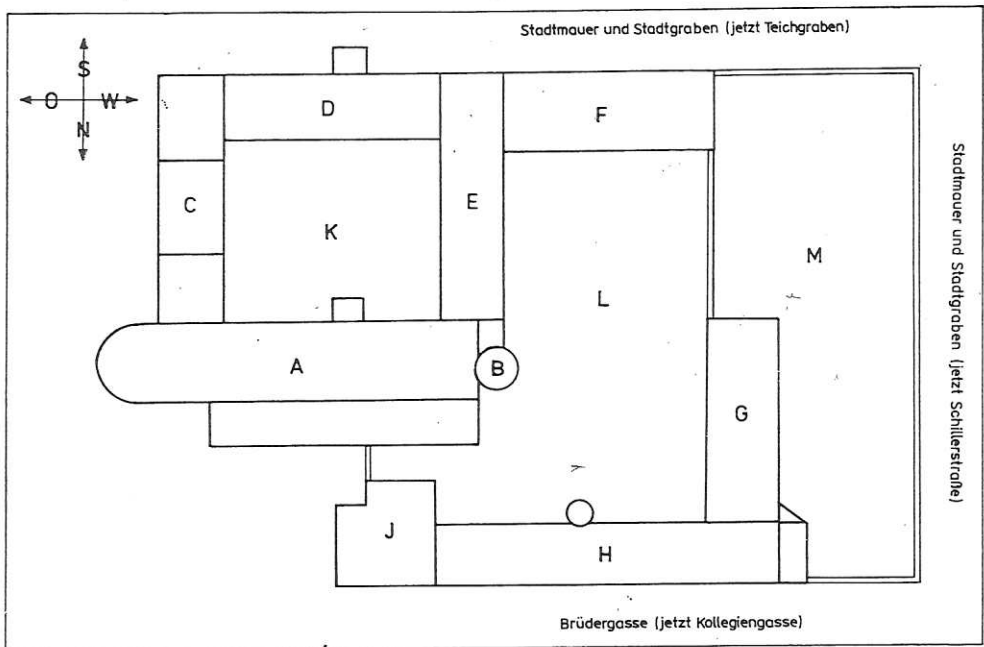
Schema zu Abb. 4—7 Grundriß des Collegium Jenense von 1557 (Aufnahmen Peter Michaelis)
